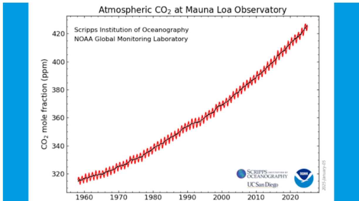
CO 2 Gehalt der Atmosphäre, gemessen seit 1960 am Mauna Loa Observatorium, Hawaii. Quellen: ->5, 3
